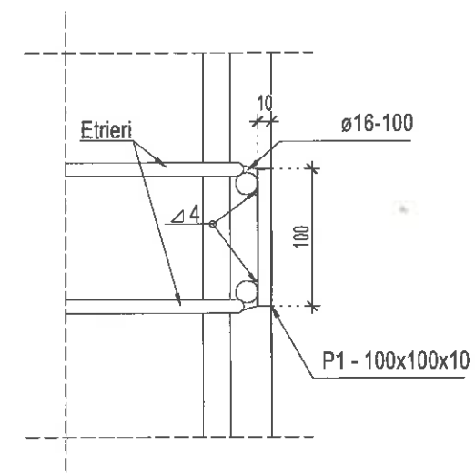
SECTIUNEA 1
