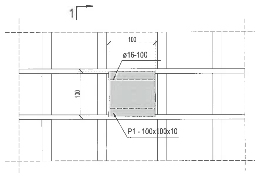
VEDERE LATERALA
