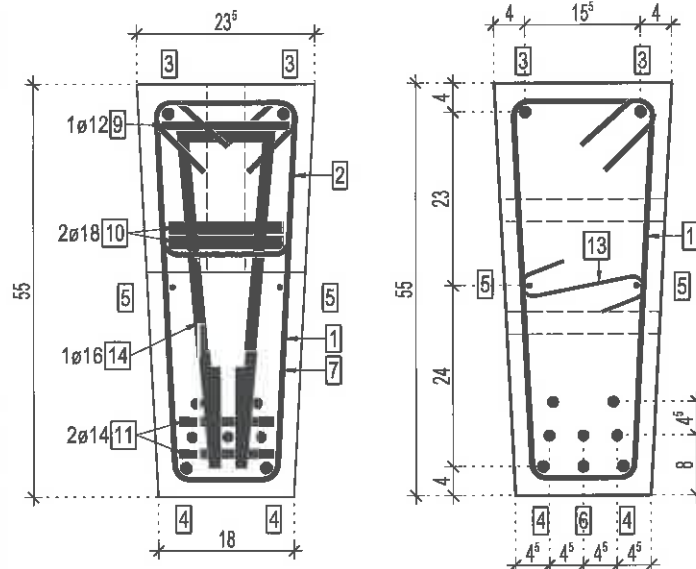
VEDEREA A-A
