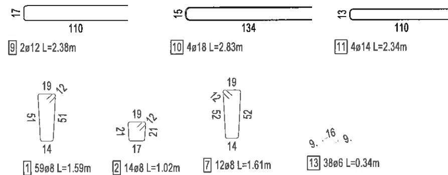
SECTIUNEA 1-1
