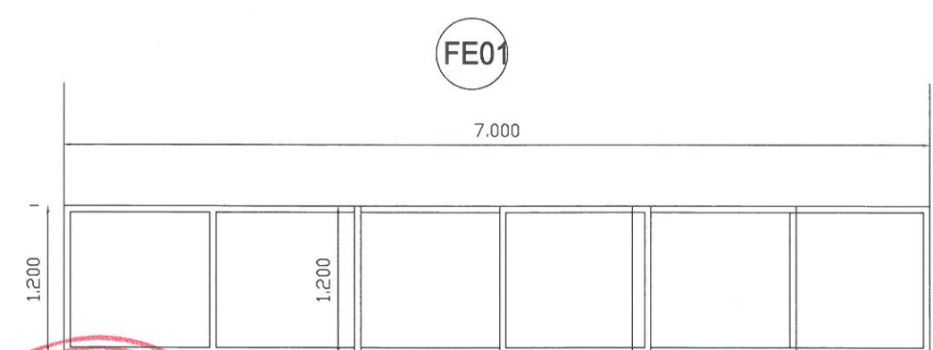
Fereastră tamplarie aluminiu RAL3001 cu geam termopan clar Deschidere: fereastră fixă UEI15-c Nr. bucati: 1
