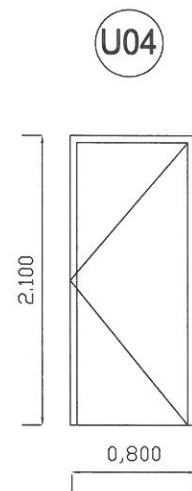
Usa din elemente metalice galvanizate RAL9002 Usa Ei30-c cu mecanism de autoinchidere Deschidere: dreapta UEI15-c Nr. bucati: 5
