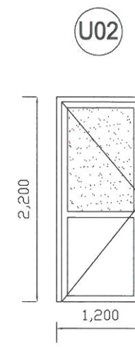
Usa tamplarie Al cu geam termopan clar RAL9002 Usa deschidere simpla Deschidere: stanga Ei15 UEI15-c Nr. bucati: 6
