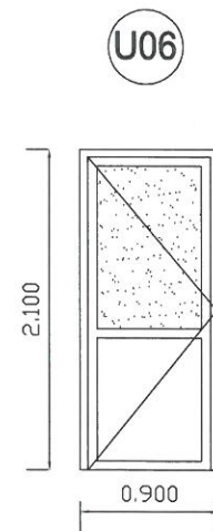
Usa tamplarie metalica RAL9002 Usa deschidere simpla Deschidere: dreapta Ei60-c UEI180-c Nr. bucati: 2
