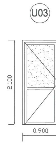
Usa tamplarie metalica cu geam termopan clar RAL9002 Usa deschidere simpla Deschidere: dreapta Ei60-c UEI120-c Nr. bucati: 2
