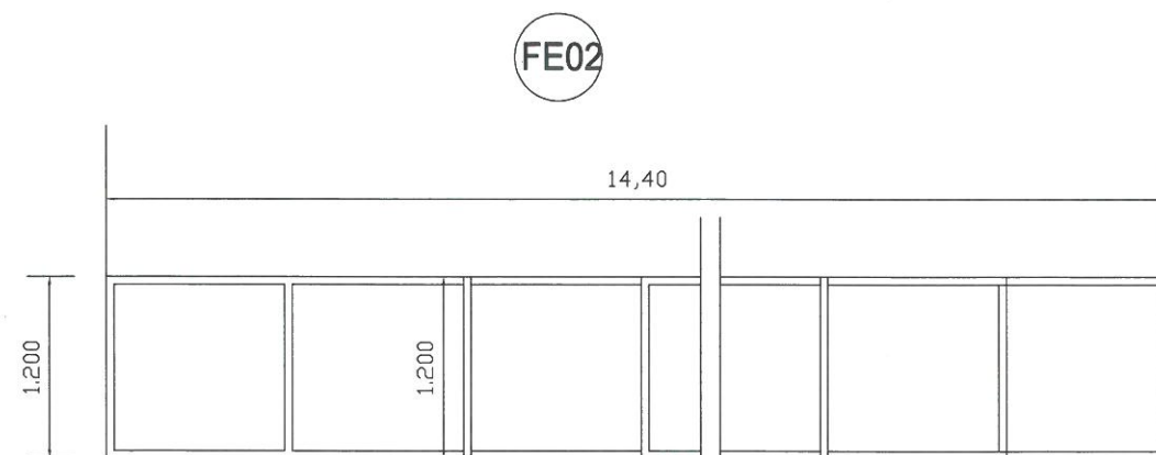
Fereastră tamplarie aluminiu RAL3001 cu geam termopan clar Deschidere: fereastră fixă UEI15-c Nr. bucati: 1
