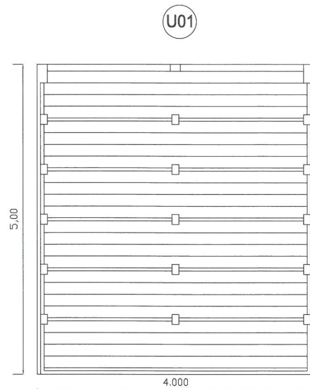
Usa sectionale cu panouri din tabla oteloasa RAL9002 Deschidere: verticala UEI15-c Nr. bucati: 4
